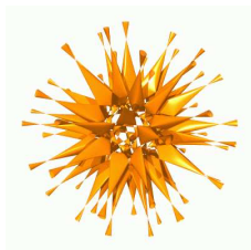
DECIC
