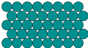
Figure 2 : assemblage hexagonal de disques dans le plan (densité \frac{\pi}{2\sqrt{3}} \simeq 0,9069 ).
