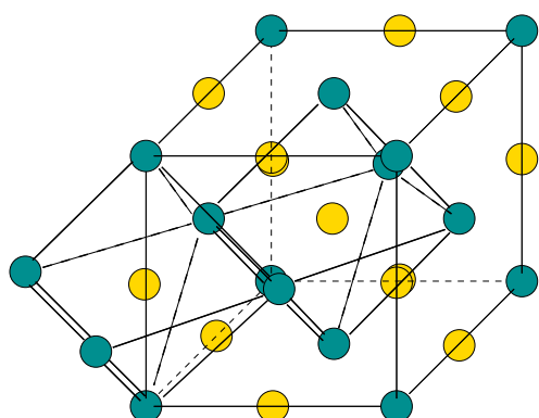
Figure 4 : sites octaédriques du réseau cubique à faces centrées, et réseau laminé en dimension 4.
