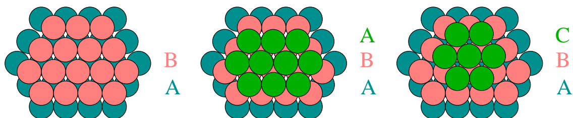
Figure 3 : empilement de couches hexagonales successives dans l'espace.
